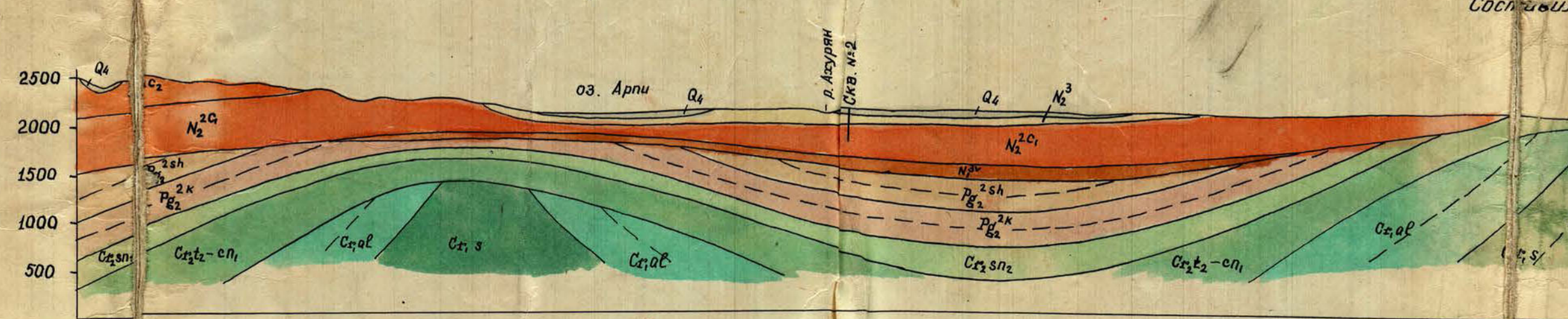
Разрез по линии А-А'
