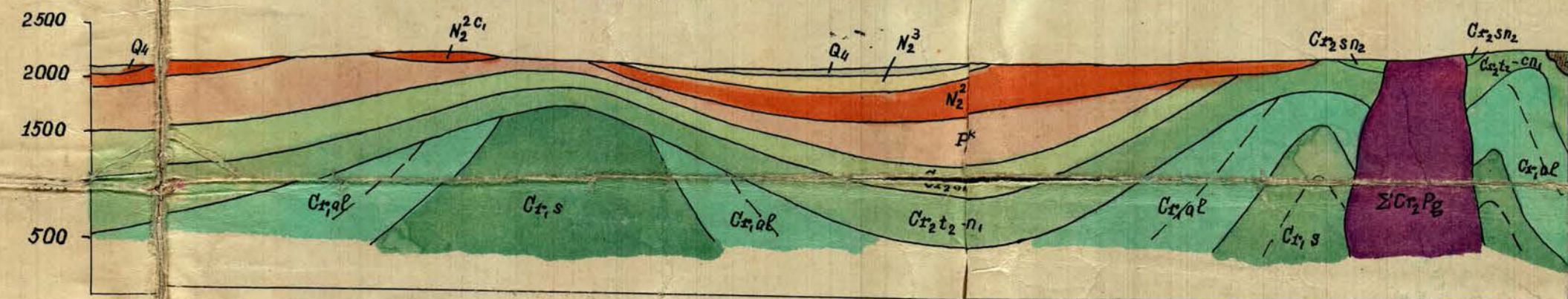
Разрез по линии Б-Б'
