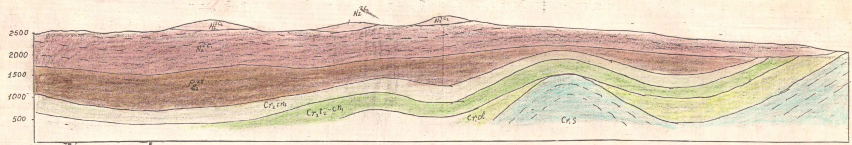
Разрез по линии А-А'
