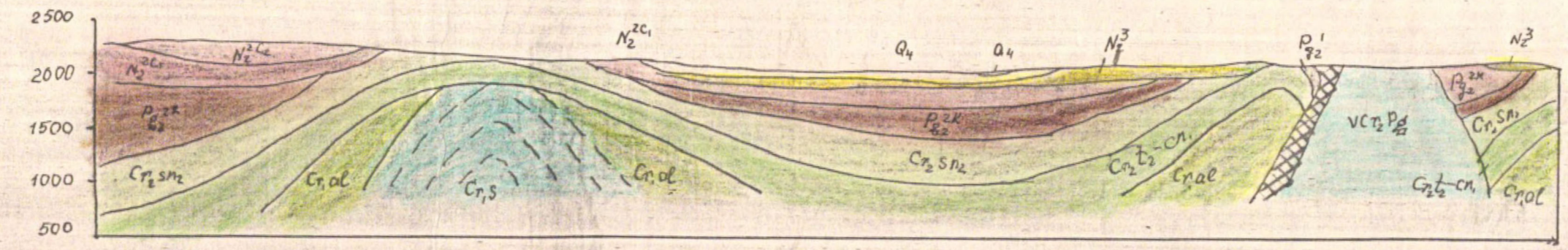
Разрез по линии Б-Б'
